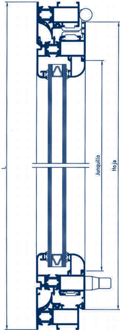
SECCION A - A
