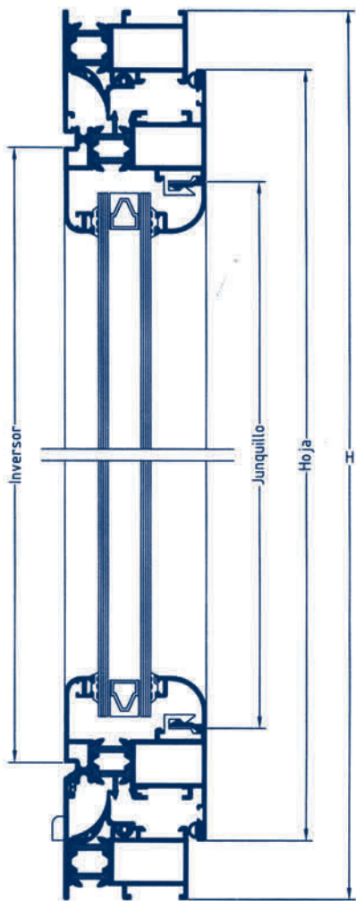
SECCION B - B
