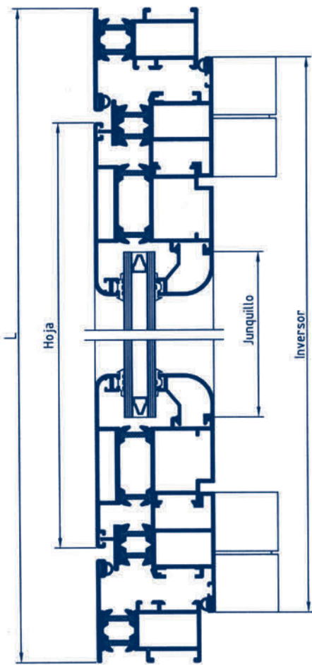
SECCION A - A
