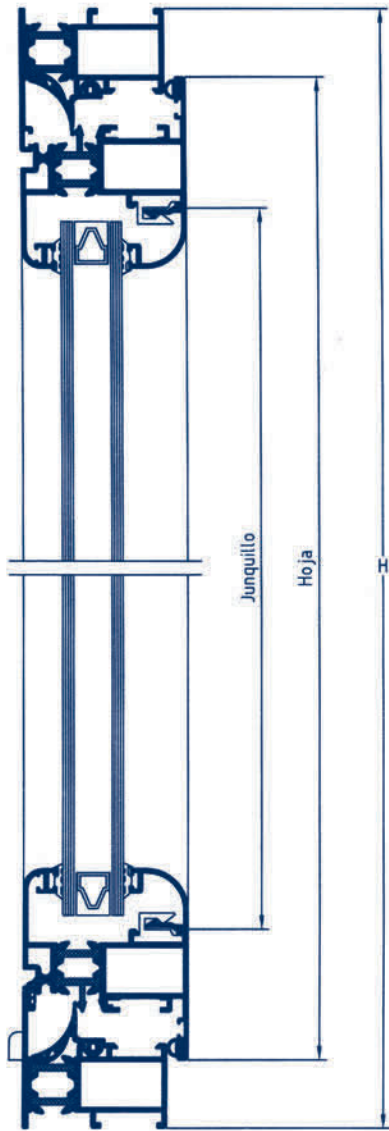
SECCION B - B
