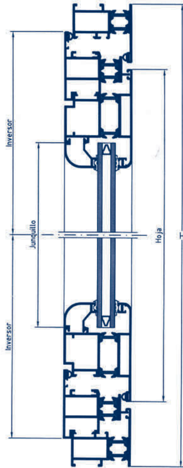
SECCION B - B
