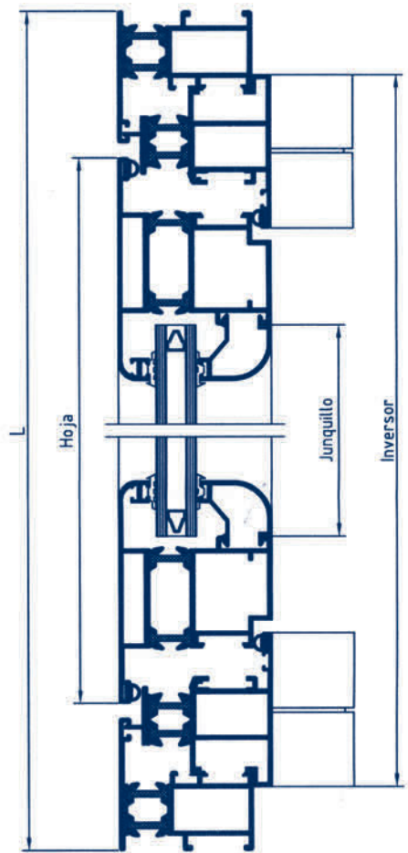
SECCION C - C
